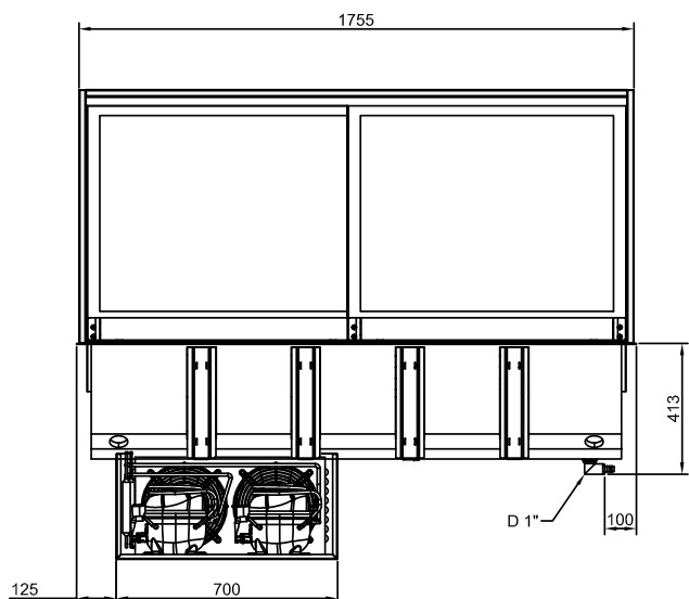
Zij aanzicht
